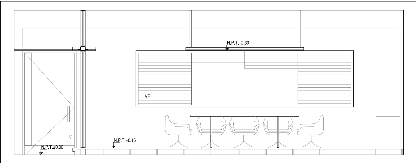
SECCIÓN B-B 1/50
