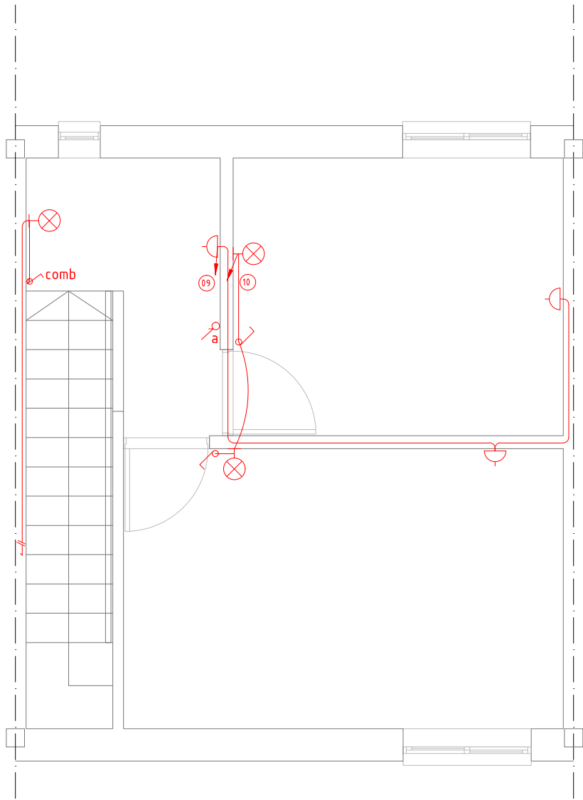
PLANTA ALTA
