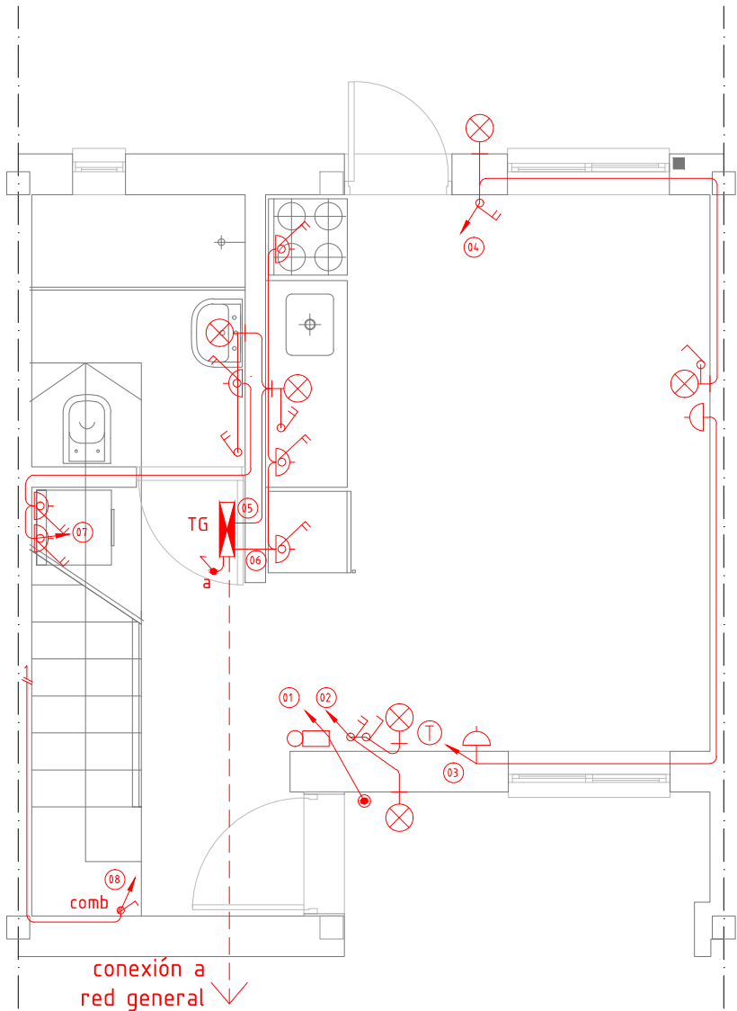
PLANTA BAJA
