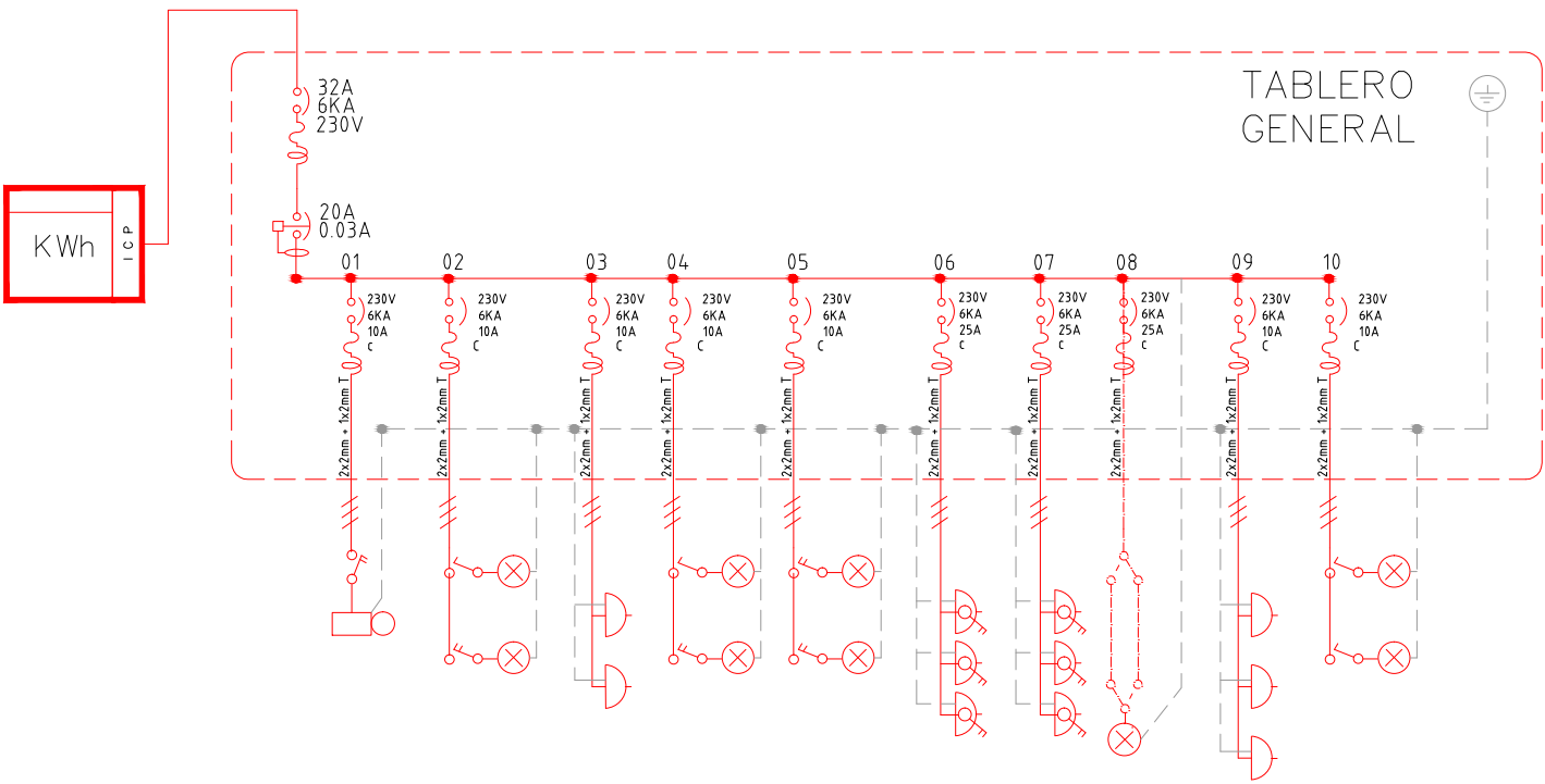
ESQUEMA UNIFILAR
