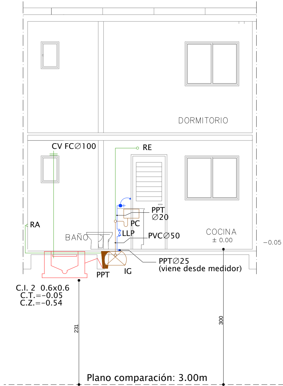
CORTE TRANSVERSAL
