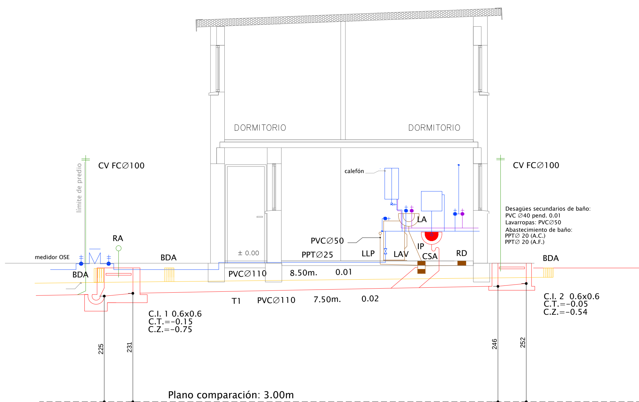
CORTE LONGITUDINAL
