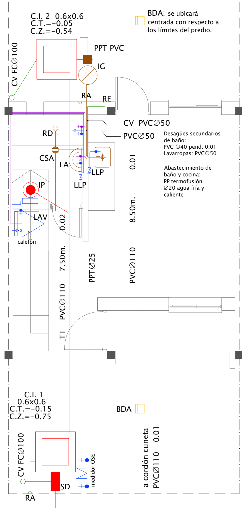
PLANTA BAJA
