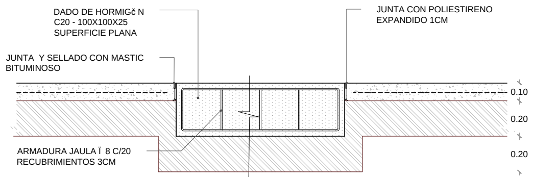
DETALLE CIMENTACION
