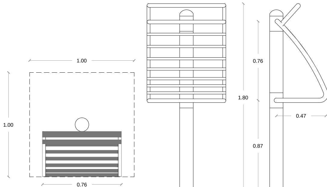
PLANTA ESQUEMA
