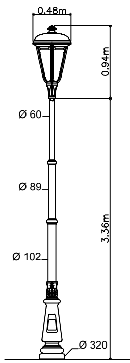
⊗ C1F DETALLE FAROLA ESC.: 1:50 CANTIDAD=102
