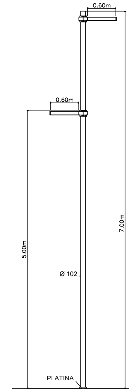
⊗ C4F DETALLE LUMINARIA ESC.: 1:50 CANTIDAD=28
